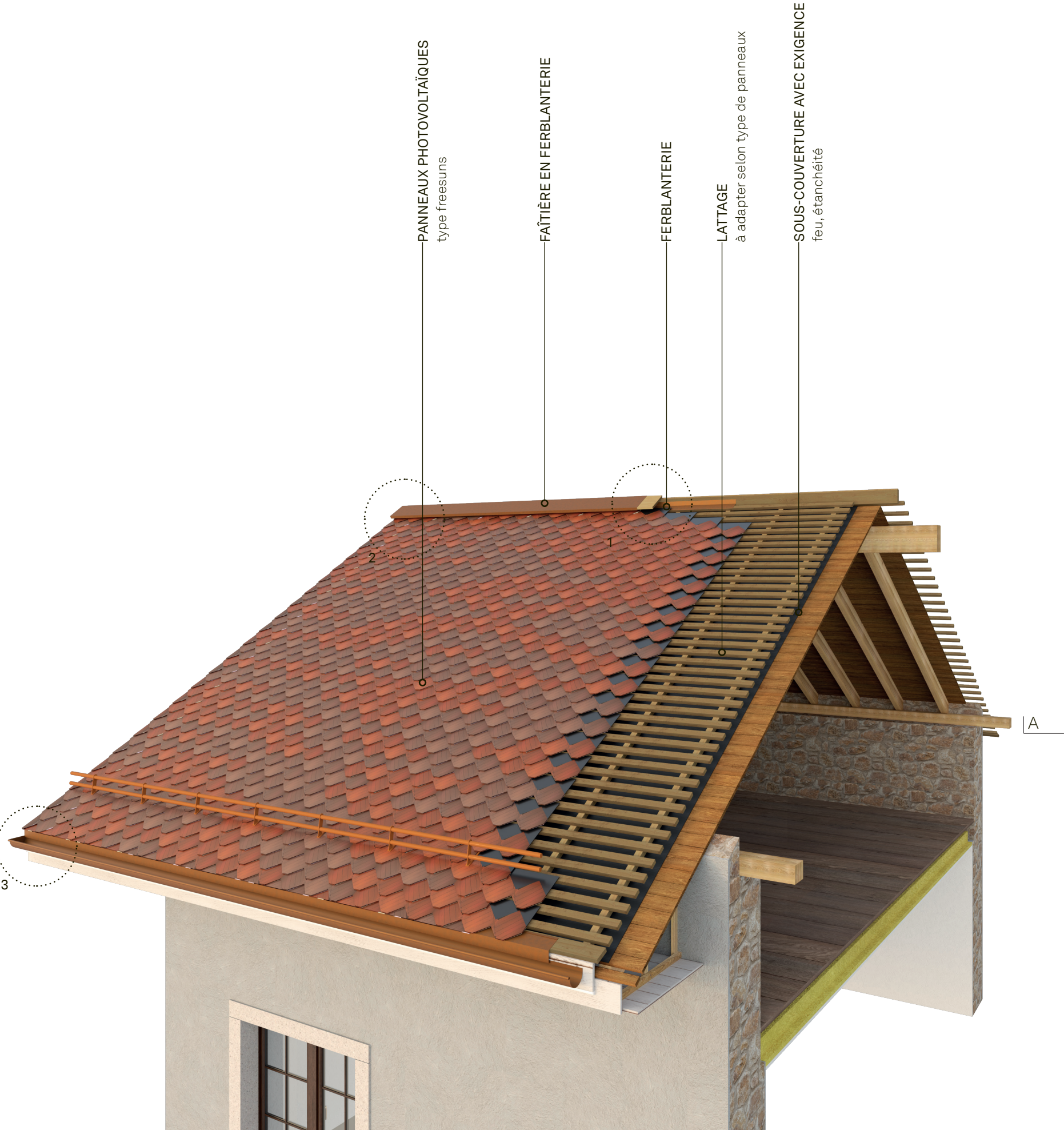
axonométrie
