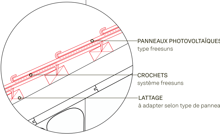
détail, échelle 1:5
