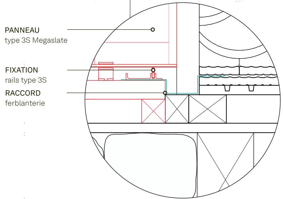
détail, échelle 1:5
