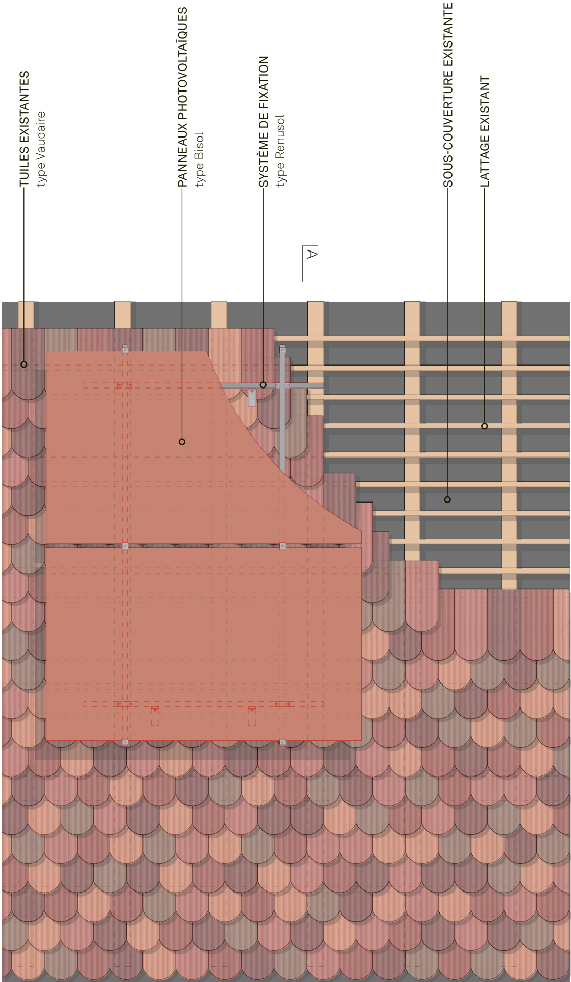
plan, échelle 1:20
