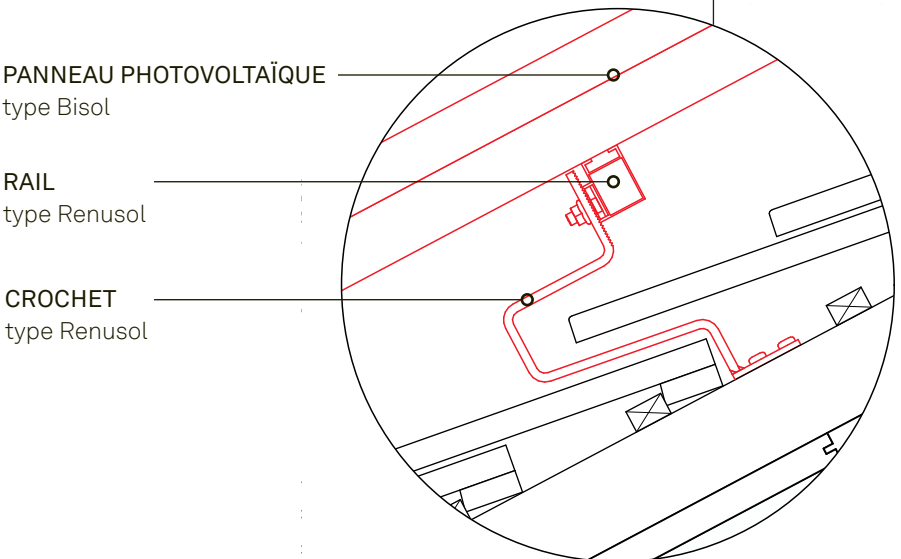
détail, échelle 1:5
