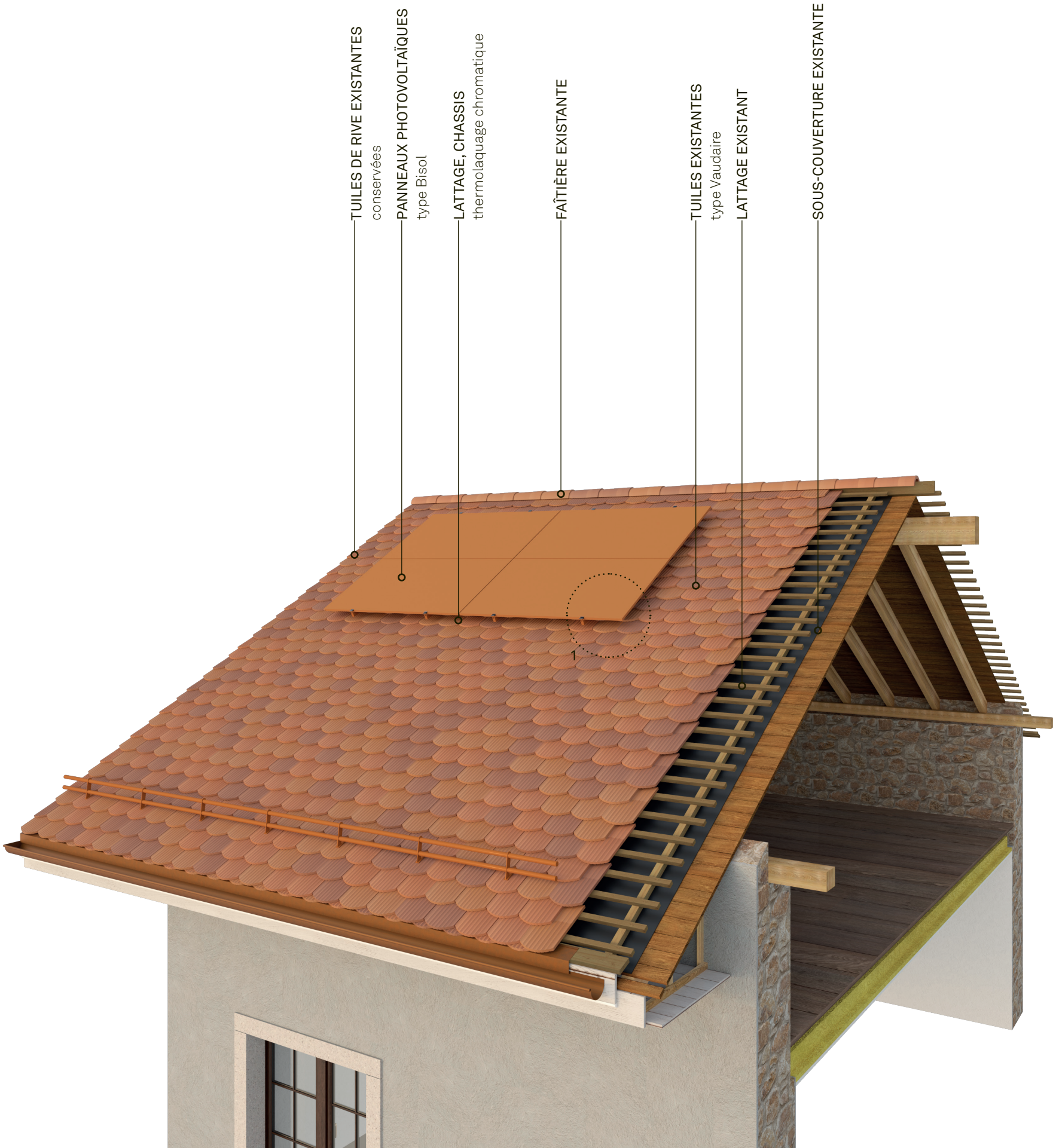
axonométrie
