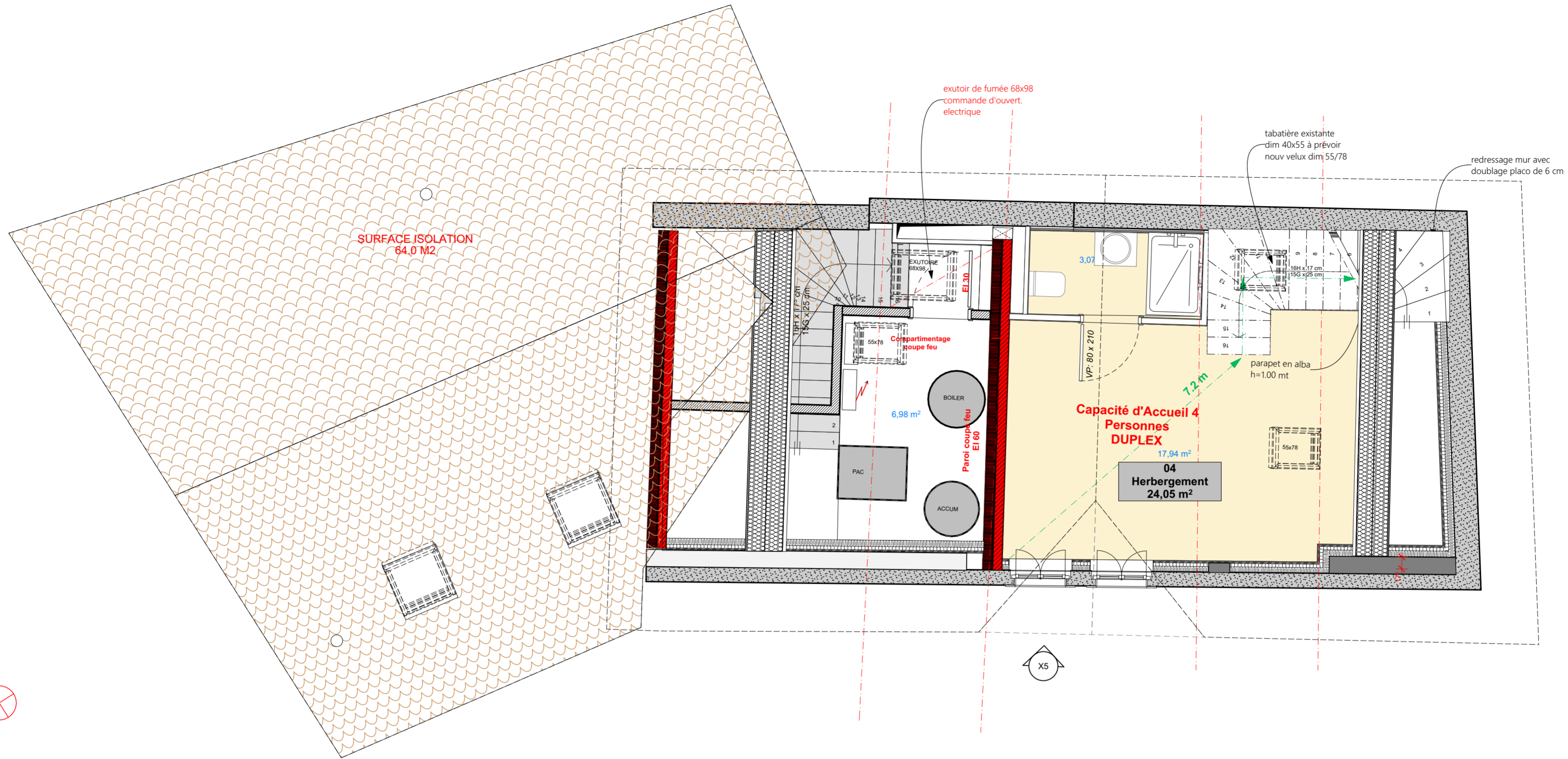
3. combles 1:50
